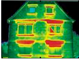
Wärmeverlust durch den Rollladenkasten
